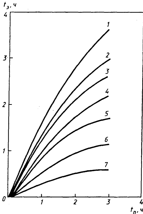
Рисунок Л.5 — Зависимость эквивалентной продолжительности пожара t_3 от продолжительности пожара t_n для горизонтальных незащищенных металлических конструкций
