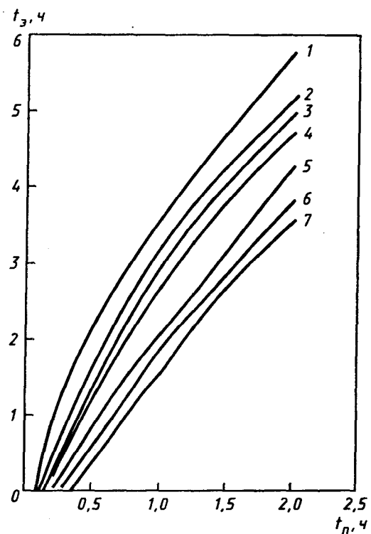
продолжительности пожара t_3 от продолжительности пожара t_n для вертикальных незащищенных металлических конструкций
